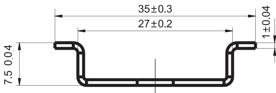
图5 安装轨尺寸
